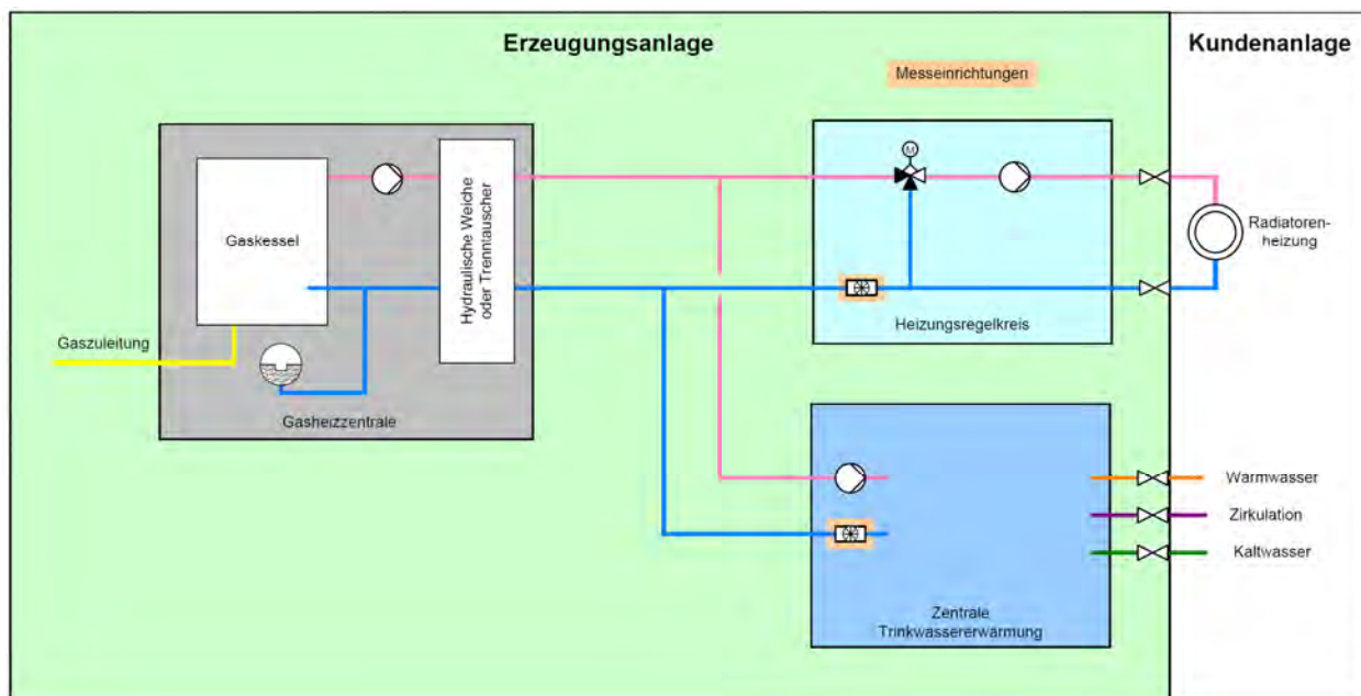
Abbildung 1: Prinzipschema Erzeugungsanlage
