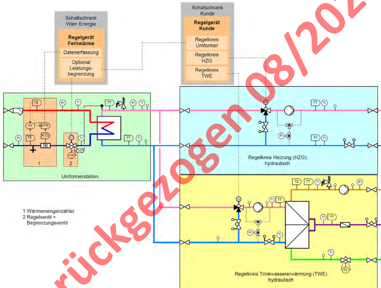
Abbildung 7: Fernwärmeregulation bei Versorgung aus dem Primärnetz bei kundeneigener Regelung
