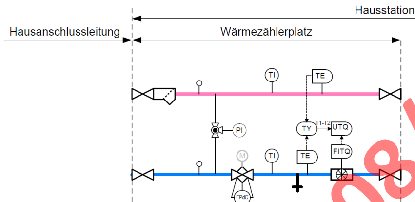
Abbildung 7: Wärmezählerplatz bei Hausstation mit mehreren Regelkreisen
