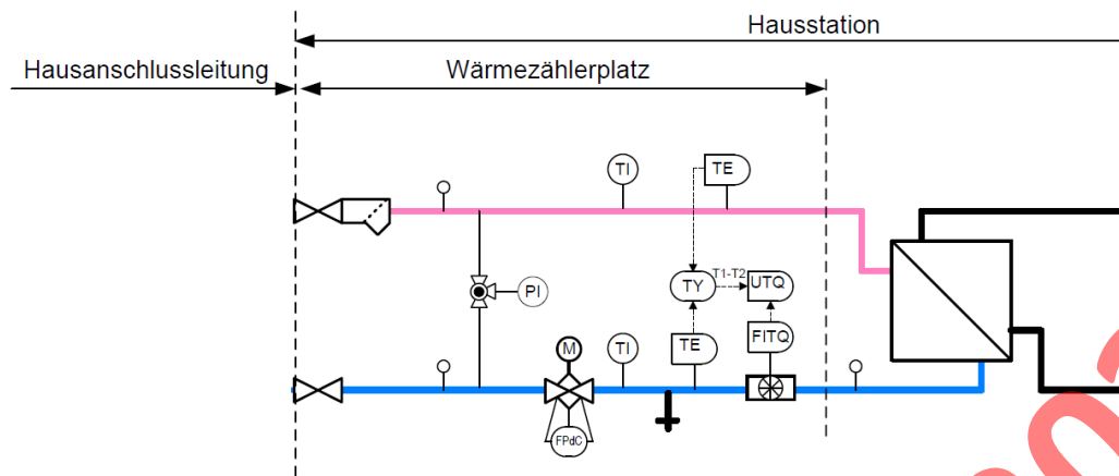
Abbildung 8: Wärmezählerplatz mit Kombiventil
