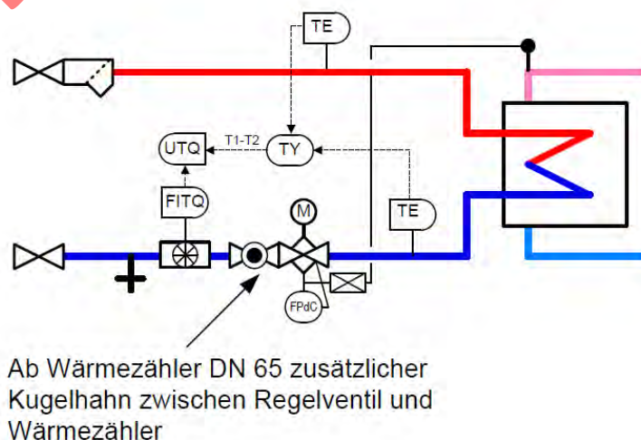
Abbildung 3: Zusätzlicher Kugelhahn bei Wärmezählern
