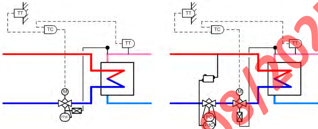
Abbildung 4: Einsatzarten von primären Regelventilen
