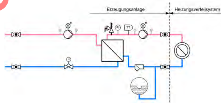
Abbildung 5: Prinzipschema Regelkreis FBH mit Trenntauscher und Drosselschaltung
