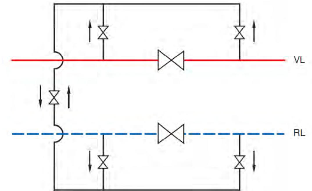
Abbildung 2 „Regelschema für H-Schaltung“
